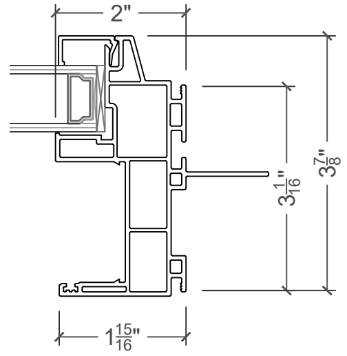
5 Jamb Detail
