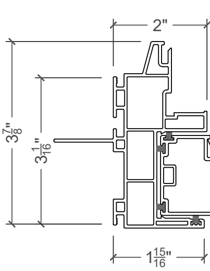
3 Jamb Detail
